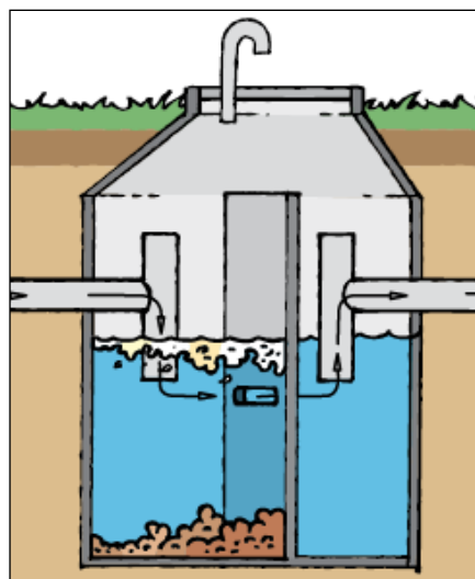
Figur 1 – Bundfældningstank
